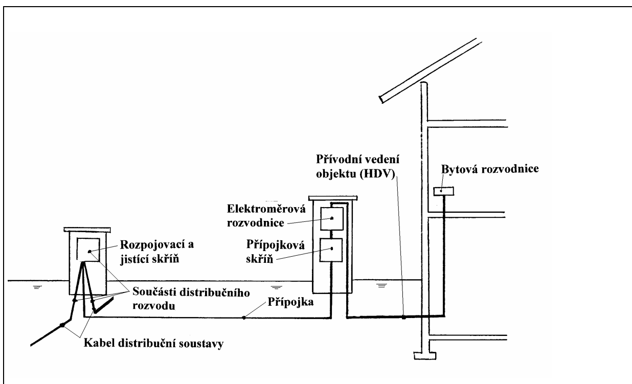
Obr. 3 Příklad připojení objektu pomocí přípojky od distribučního kabelového vedení z rozpojovací jistící skříně
