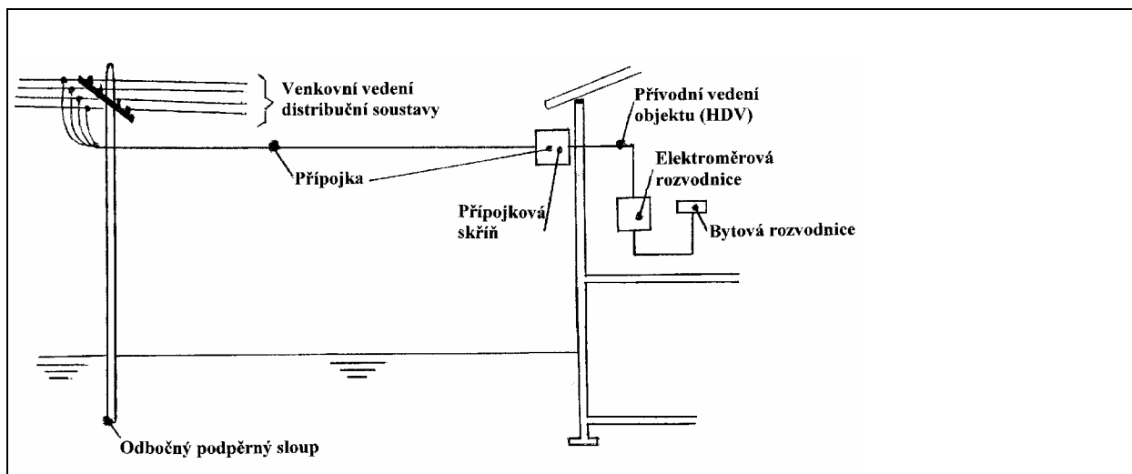
Obr. 1 Příklad připojení objektu pomocí přípojky provedené venkovním vedením od distribučního venkovního vedení (místo samostatných vodičů venkovního distribučního vedení může být užito i zavěšeného (závěsného) kabelu) Poznámka: přívodní vedení objektu v tomto případě může být považováno i za odbočku k elektroměru)
