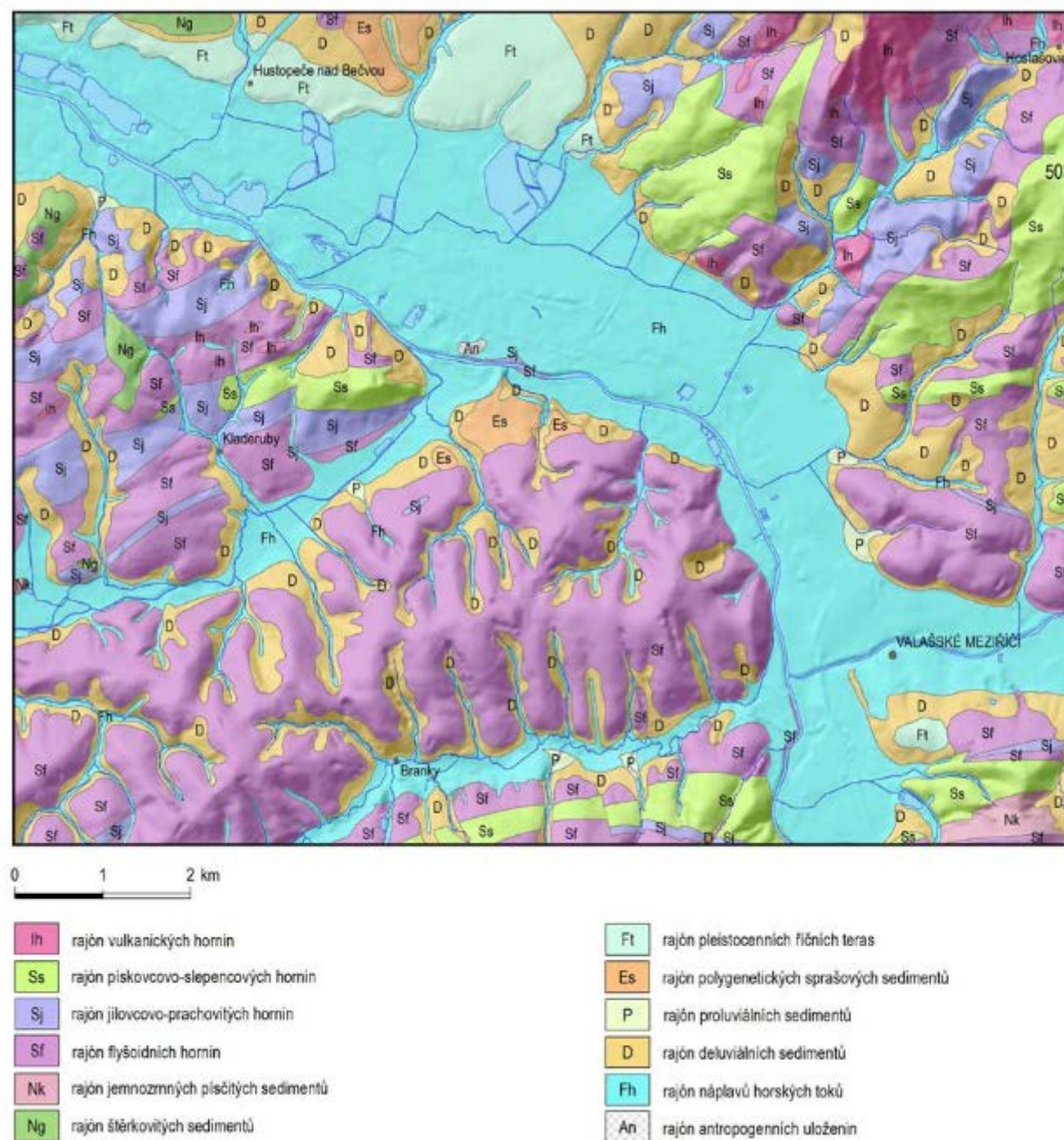
Obr. 2: Schématická mapa inženýrskogeologických rajónů předkvartérních a kvartérních hornin a zemin zájmového území plánovaného VD Skalička.
