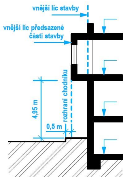
ŘEZ
