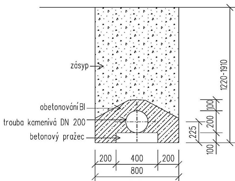
PŘÍČNÝ ŘEZ
