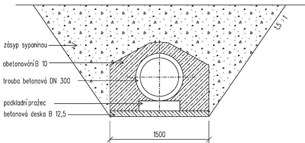
PŘÍČNÝ ŘEZ
