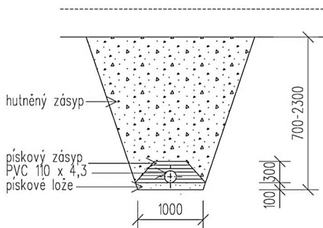
PŘÍČNÝ ŘEZ
