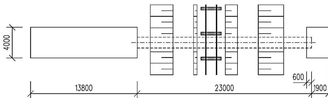
PŮDORYS
