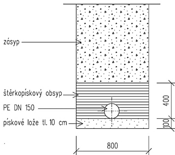
PŘÍČNÝ ŘEZ
