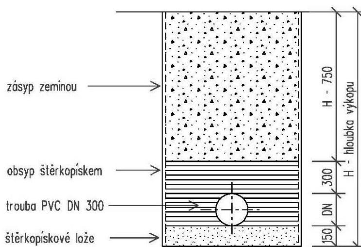
PŘÍČNÝ ŘEZ
