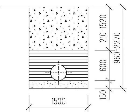
PŘÍČNÝ ŘEZ
