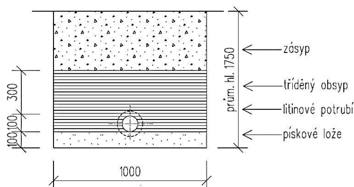
PŘÍČNÝ ŘEZ
