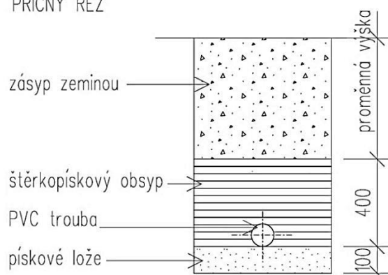
PŘÍČNÝ ŘEZ
