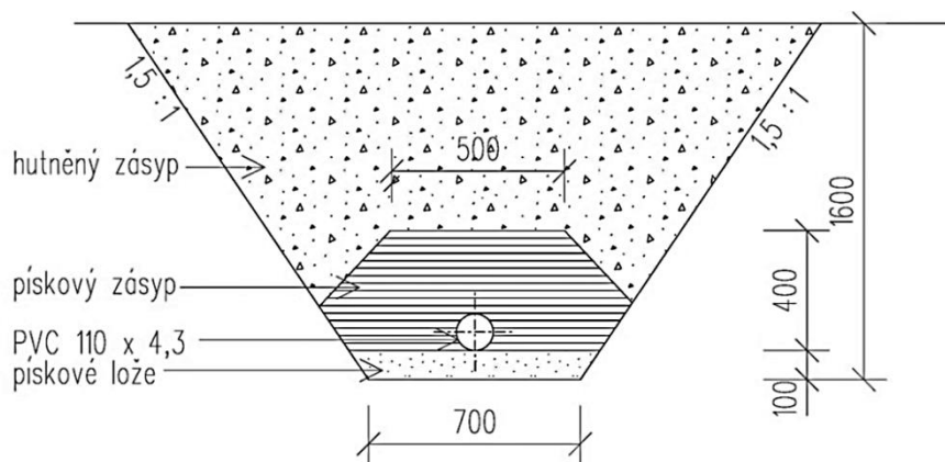
PŘÍČNÝ ŘEZ
