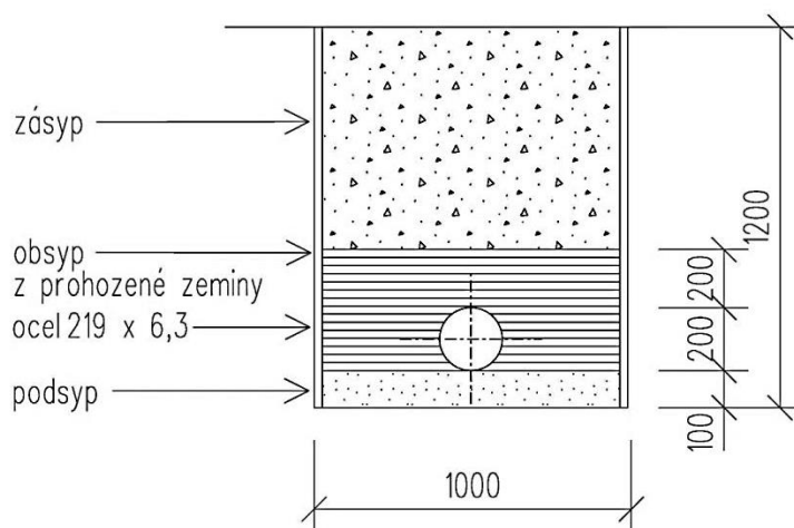
PŘÍČNÝ ŘEZ
