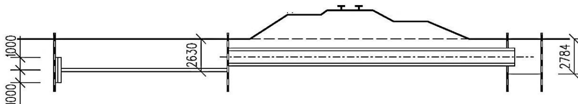
PODÉLNÝ ŘEZ
