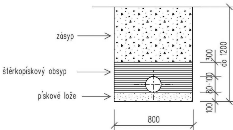
PŘÍČNÝ ŘEZ
